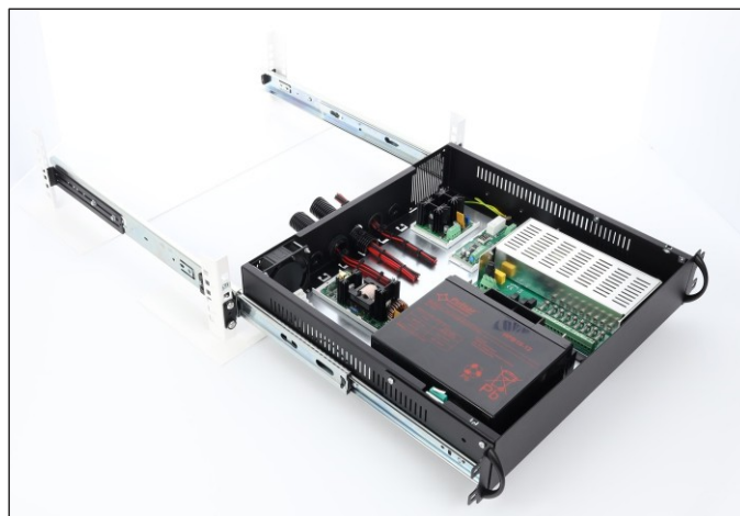
Skriňu s posuvníkmi zasunúť do koľajníc nainštalovaných v 19" skrini RACK
