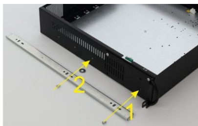
Pripevnite jazdce dvoma skrulkami ku skrini ARAD (nezabudnite na dištančnú podložku pod druhou skrulkou).
