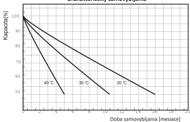
Charakteristiky samovybíjania
