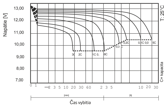
Charakteristiky vypúšťania
