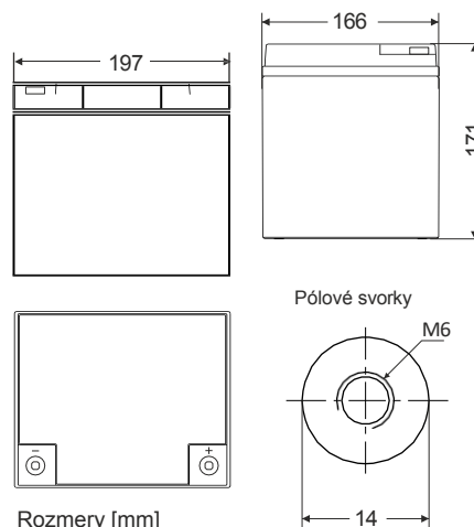
Rozmery [mm] Tolerancia: Tolerancia: +/- 2 mm;
