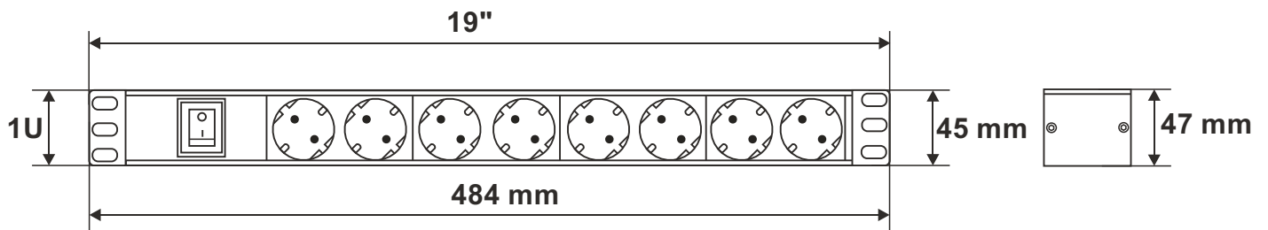
plug: type: E/F („Unischuko”)
