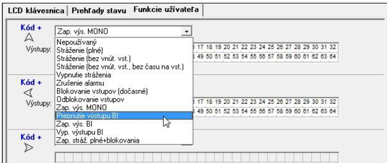
Obr. 10. Záložka „Funkcie užívateľa“ pre LCD klávesnicu v programe DLOADX.
