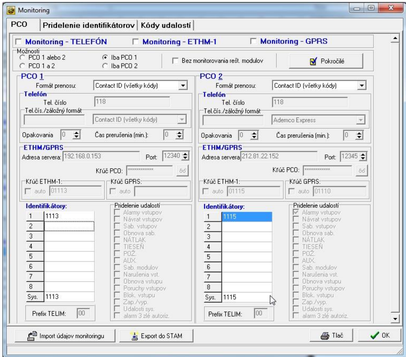
Obr. 11. Príklad nastavení monitoringu v programe DLOADX.
