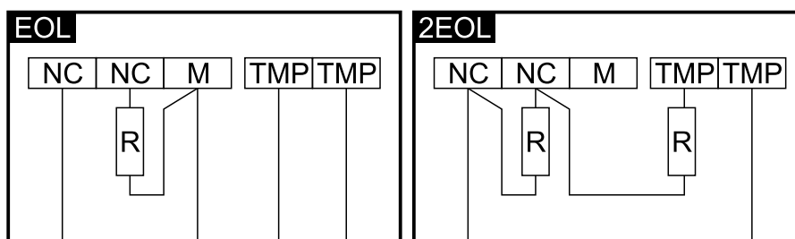
Obr. 1. Spôsob pripojenia vodičov a rezistorov pre konfiguráciu EOL a 2EOL.
